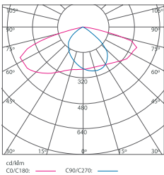
ECO MINI 12W (200W)
