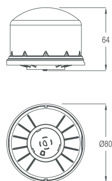
LCU ZHAGA WiSZ SOLAR Z10
