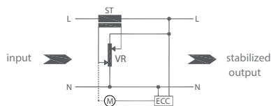
single phase avs / avr
