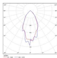
CDM-T 70W G12
